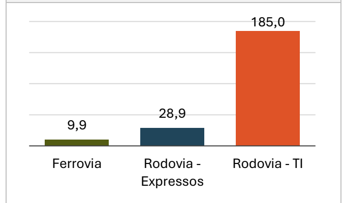
Figura 21 – Custos com a energia de tração por 1000 PKm (Fonte: AMT)
