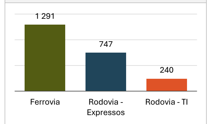
Figura 19 – Custos com a energia de tração por veículo e por 1000 km (Fonte: AMT)
