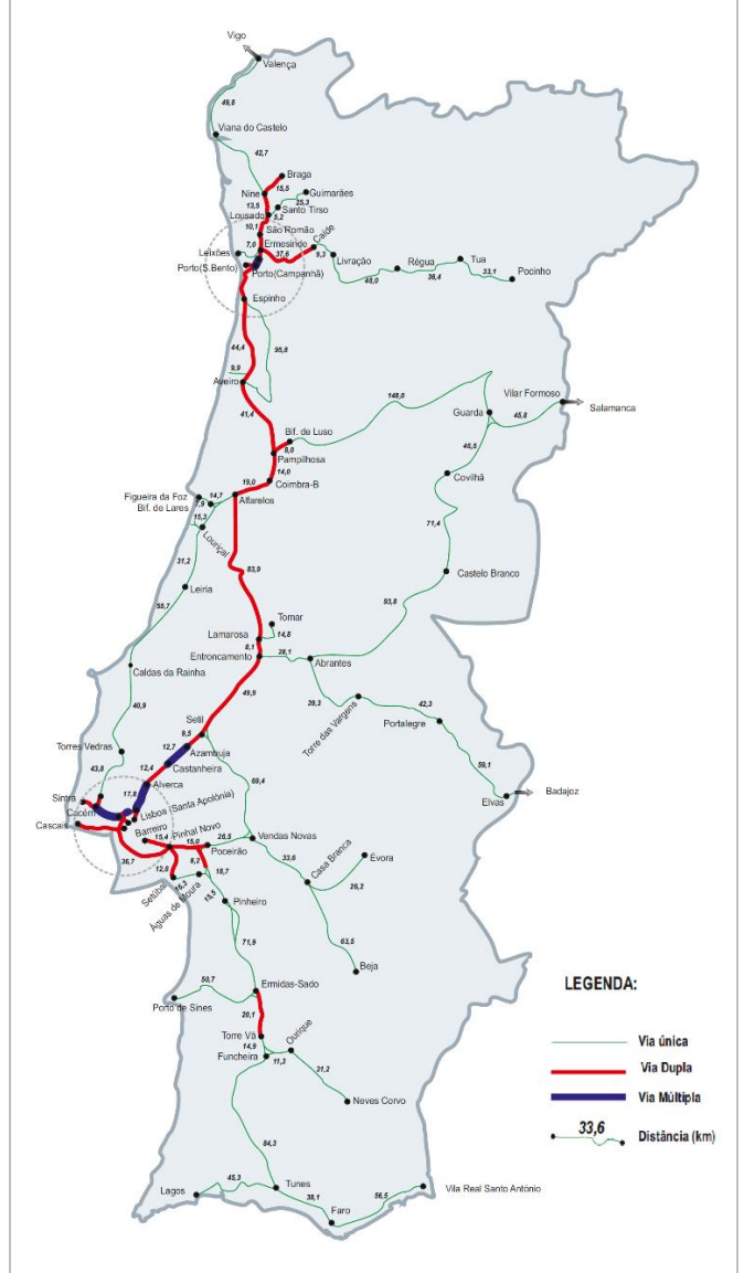
Figura 9 – Mapa da RFN por tipologia das vias e distâncias (Fonte: Diretório da Rede 2023, IP)
