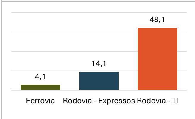
Figura 20 – Custos com a energia de tração por 1000 LKm (Fonte: AMT)
