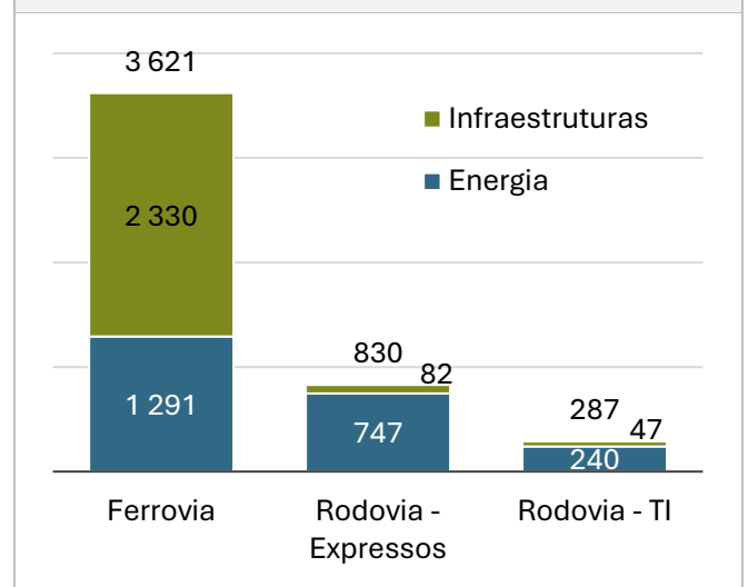
Figura 22 – Custos com o acesso à infraestrutura e com a energia de tração por veículo e por 1000 km (Fonte: AMT)
