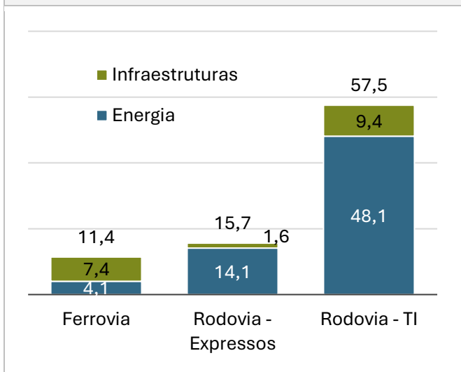
Figura 23 – Custos com o acesso à infraestrutura e com a energia de tração por 1000 LKm (Fonte: AMT)
